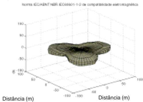
Fig. 7. Zonas de exclusão conforme a norma de compatibilidade eletromagnética. Escala = 100 m. (a) perspectiva; (b) projeção horizontal; (c) projeção vertical.
