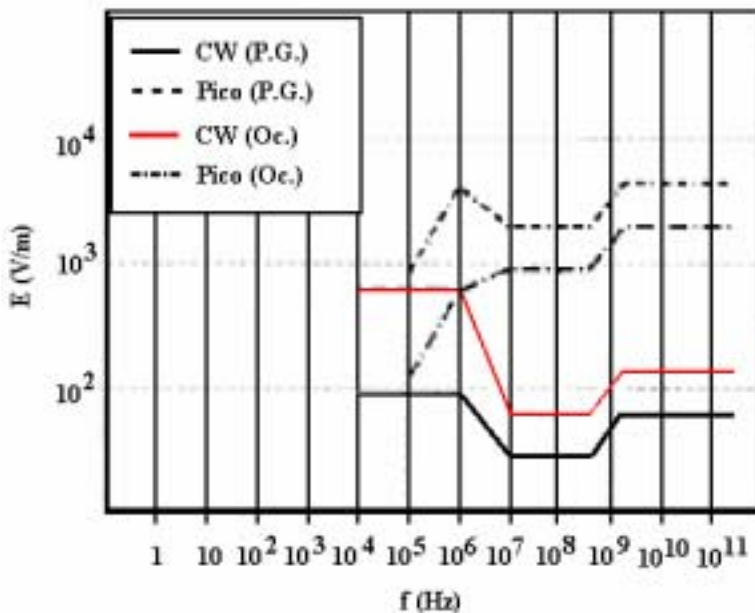
Figura 25 Limites de intensidade de campo elétrico da Resolução 303 da ANATEL.
