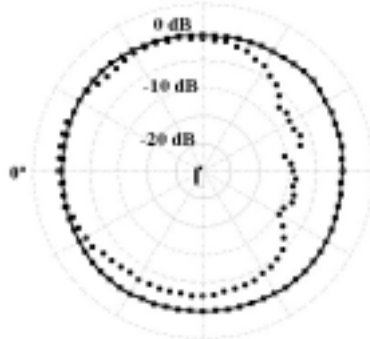
Fig. 14b. Diagrama de irradiação horizontal em espaço livre (sem a cabeça): Linha contínua → monopolo de \frac{1}{4} de onda, Linha pontilhada → antena diretiva.
