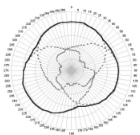
Fig. 2. Diagrama de irradiação horizontal de cada uma das antenas (linhas tracejadas) e o valor do somatório obtido (linha contínua).
