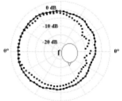
Fig. 14c. Diagrama de irradiação horizontal na situação de uso (com a cabeça): Linha contínua → monopolo de \frac{1}{4} de onda, Linha pontilhada → antena diretiva.
