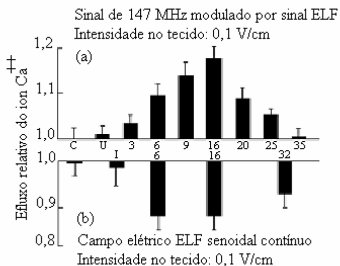
Figura 18 (a) Efluxo do íon Ca ++ por um sinal de 47 MHz modulado por um sinal ELF; (b) por um sinal ELF contínuo.
