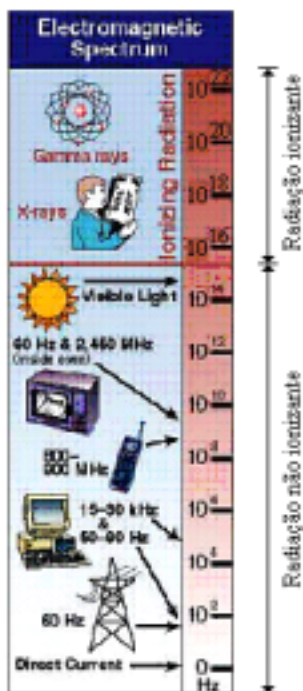
Figura 9 Espectro eletromagnético simplificado.
