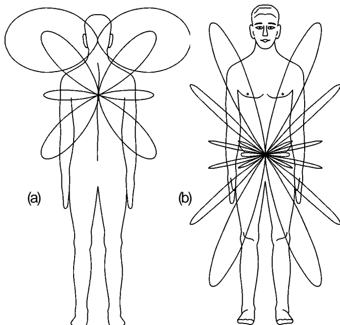
Figura 1(a-b) Lóbulos de absorção de um ser humano na frequência de 825 MHz, considerando (a) o sistema nervoso central (liquor encefalo-raquiano) e a caixa craniana ou (b) considerando o sistema circulatório (veias e artérias) ou o sistema linfático, como antenas.
