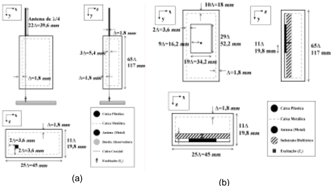
Fig. 11. (a) Representação do aparelho celular portátil modelado com antena tipo monopolo de \frac{1}{4} de onda alimentada por cabo coaxial, e (b) com antena planar com alimentador coaxial.
