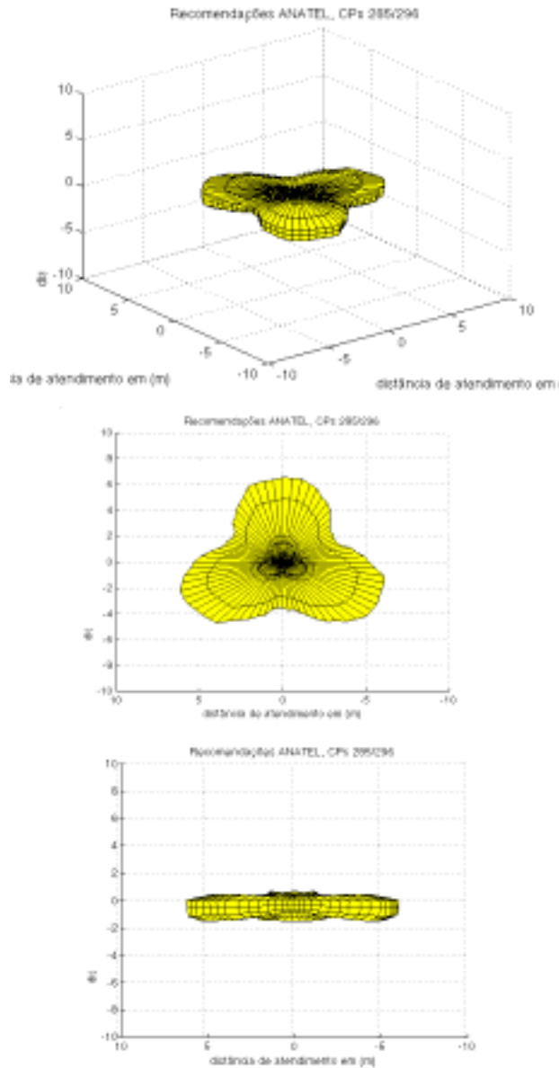
Fig. 3. Zonas de exclusão conforme a recomendação adotada pela ANATEL. Escala = 10 m. (a) perspectiva; (b) projeção horizontal; (c) projeção vertical.
