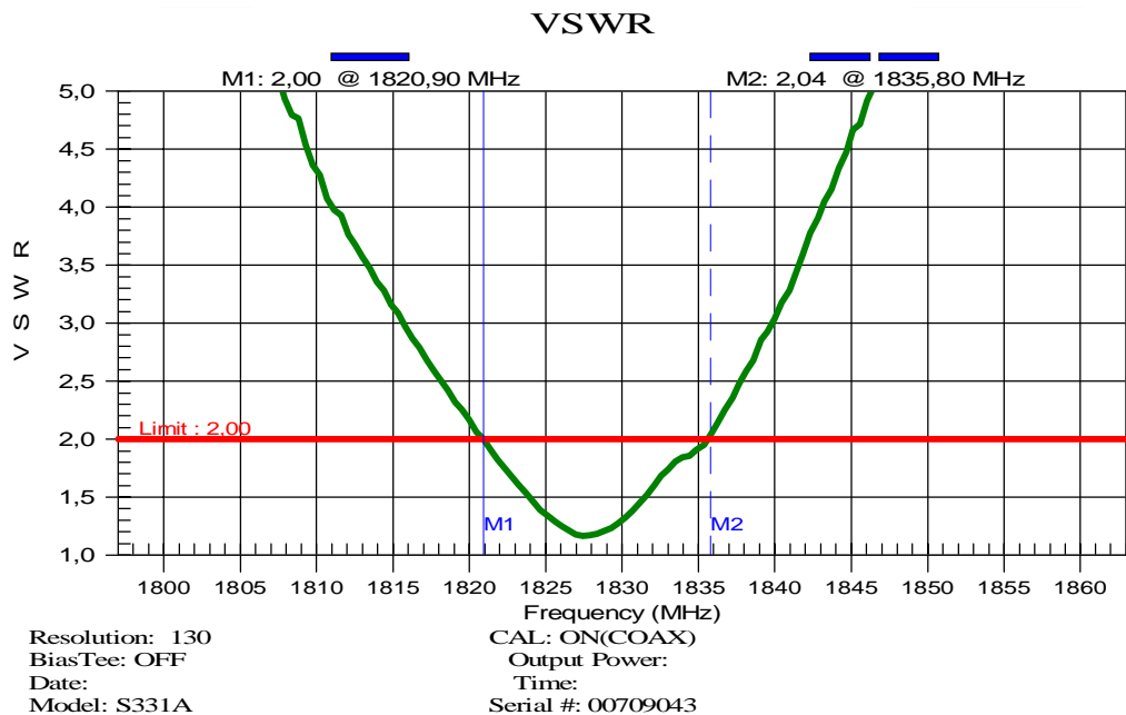
Figura 16. Taxa de onda estacionária para a antena patch : (a) simulada no Ensemble® e (b) medida com o S331A.
