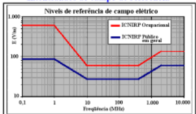
Figura 24 Limites de intensidade de campo elétrico do padrão ICNIRP.
