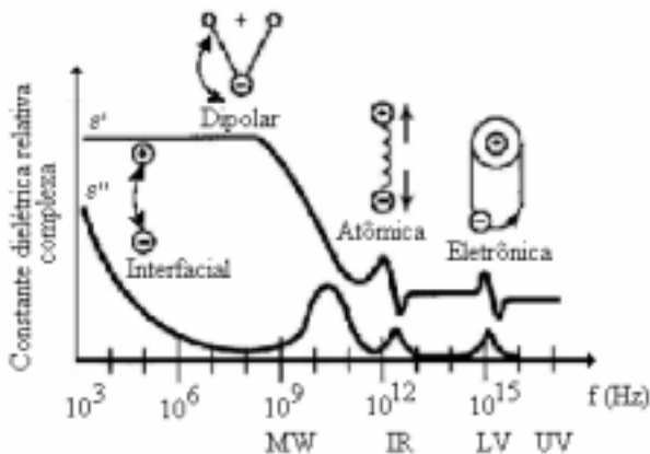
Figura 14 Diagrama de dispersão dielétrica de biomateriais.
