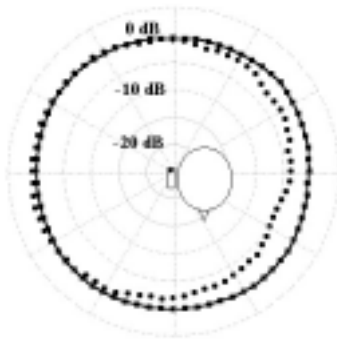
Fig. 14a. Diagrama de irradiação horizontal para a antena monopolo de \frac{1}{4} de onda: Linha contínua → sem a cabeça, Linha pontilhada → com a cabeça.
