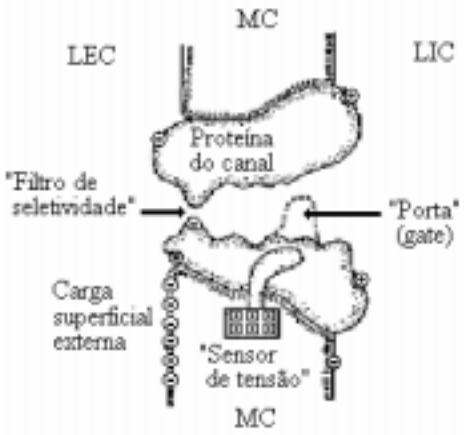
Figura 17 Canal iônico gatilhado a tensão.
