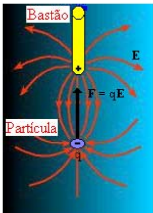
Figura 2 Força de atração entre a carga elétrica positiva de um bastão atritado e uma partícula de papel carregada negativamente.
