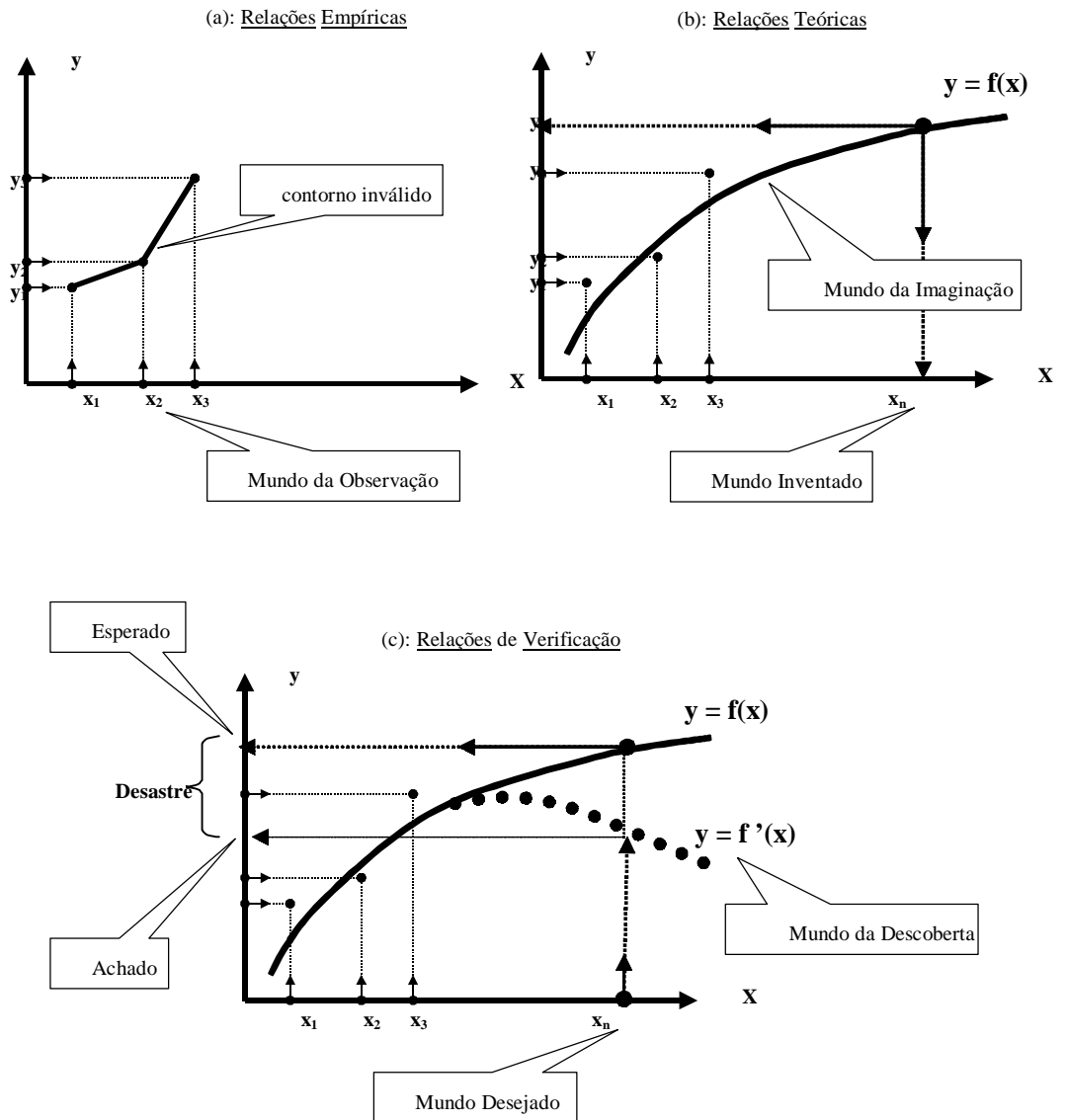
Figura 1: Processo de produção e uso do conhecimento científico. (a) As relações empíricas ( X_i e Y_i ) correspondem ao mundo observado mas não podem ser extrapoladas, pois contém o erro da observação. (b) Quando uma relação teórica é estabelecida, a extrapolação é possível porque a relação matemática é perfeita, permitindo a invenção do não existente. (c) A verificação empírica da teoria deixa explícito o mundo da descoberta. Quando o achado não confere com o esperado, configura-se o “desastre” e a relação teórica pode assumir uma nova forma, mais completa.
