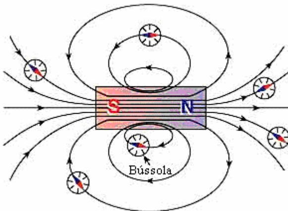
Figura 1(a) As linhas de campo magnético podem ser visualizadas por meio de uma pequena bússola. O pólo norte (azul) da agulha aponta na direção do campo magnético em qualquer ponto do campo produzido pelo ímã.
