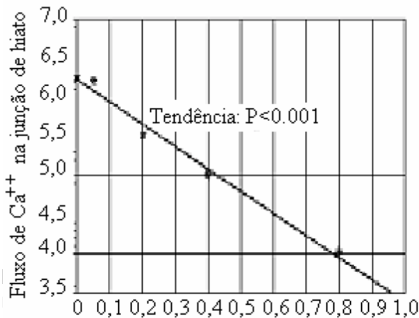
Figura 20 Fluxo de \text{Ca}^{++} na junção de hiato, em função da intensidade de campo magnético de 50 Hz. (Liu et al., 1995)
