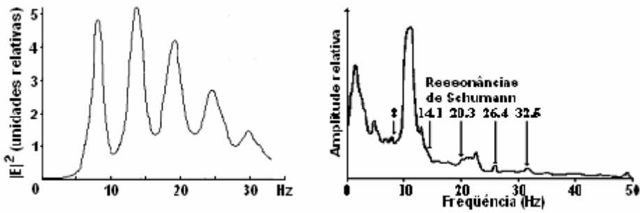
Figura 23 Ressonância de Schumann típica (esquerda) e EEG (estado de alerta) típico, com superposição dos picos de ressonância de Schumann (direita).
