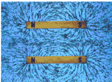
Figura 1(b) As limalhas de ferro se transformam em pequenos ímãs induzidos e sua disposição espacial descreve a configuração do campo magnético dos dois ímãs.
