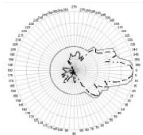
Fig. 1. Diagrama de irradiação vertical da antena (linha tracejada) e seu valor corrigido para efeitos de cálculo (linha contínua) de acordo com a norma da Suíça.
